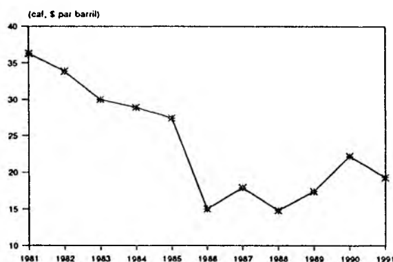
Gr. 4.5 - Prix à l'importation de l'OCDE du pétrole brut
